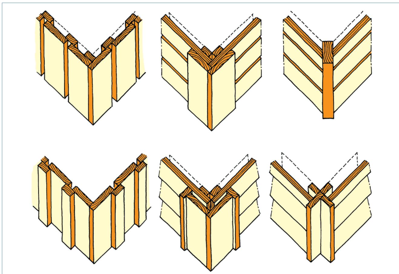
Figur 6. Hjørneløsninger for liggende kledning.
