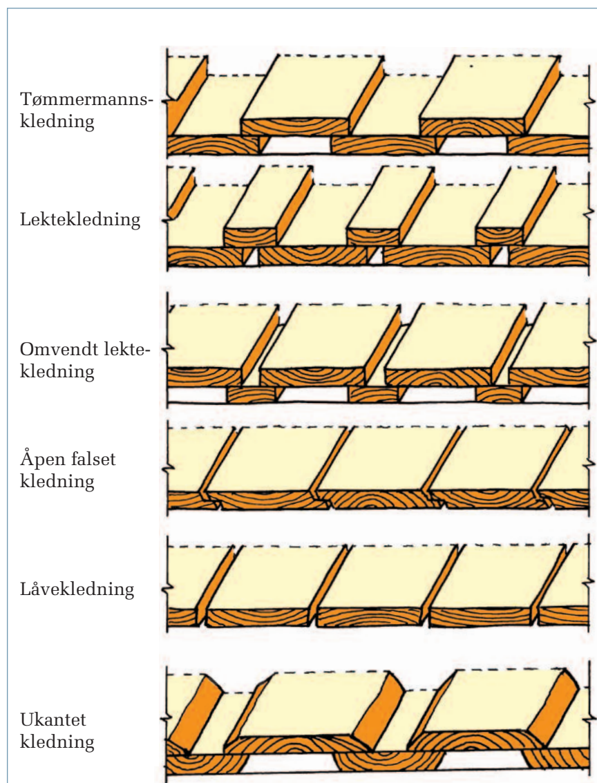
Figur 2. De vanligste typene av stående kledning.
