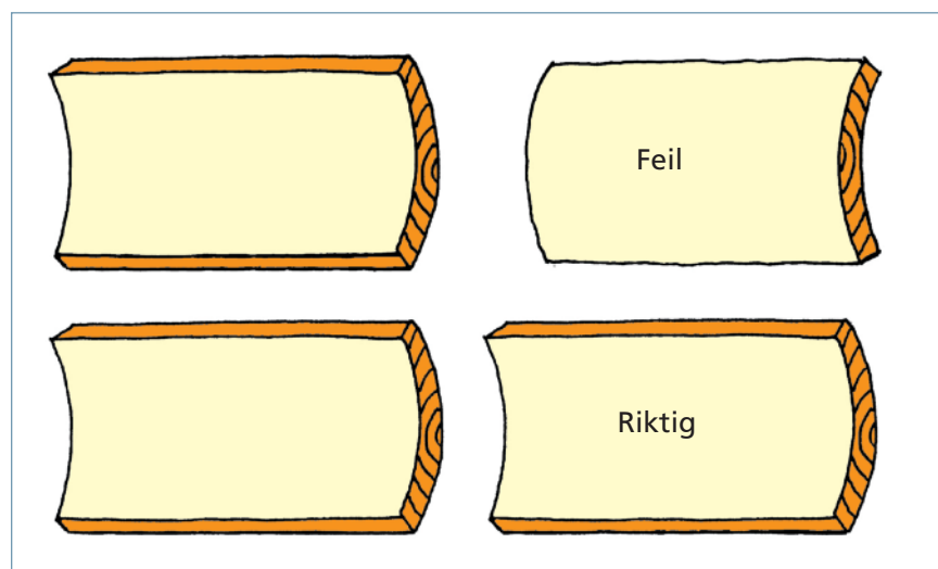
Figur 7. Det er viktig å skjøte bord med lik årringretning. (Krumning er sterkt overdrevet.)
