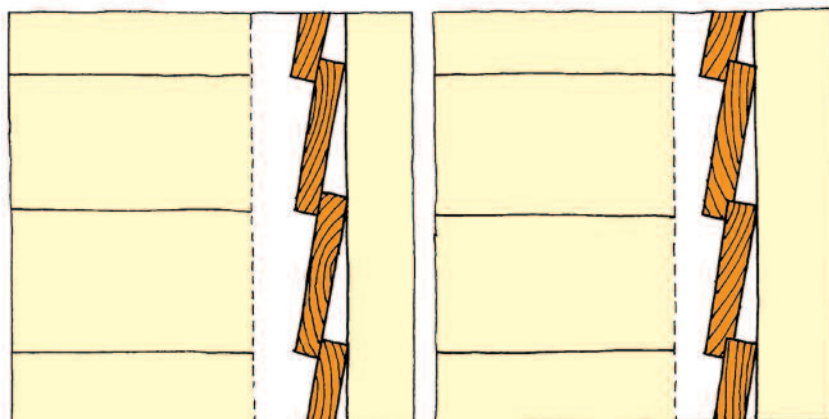
Enkel liggende kledning
